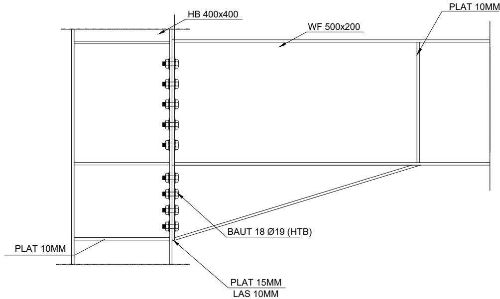
DETIL B1 KE KOLOM SKALA 1 : 15
