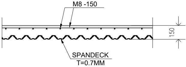
DETIL PLAT METAL DECK SKALA 1 : 25
