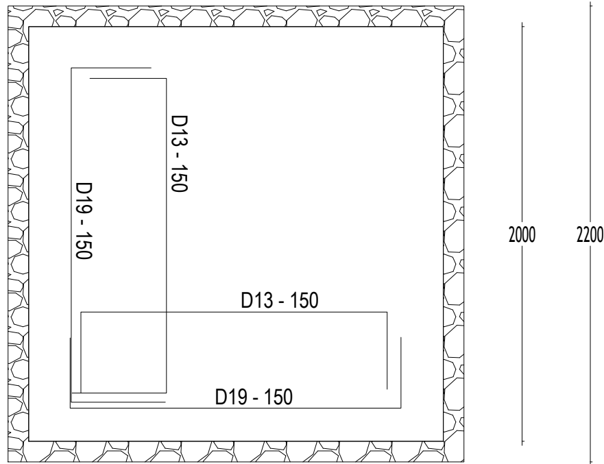
DETAIL FONDASI F2
