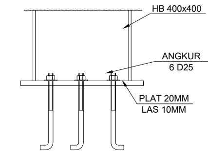
DETIL KOLOM K1 HB 400x400 SKALA 1 : 15
