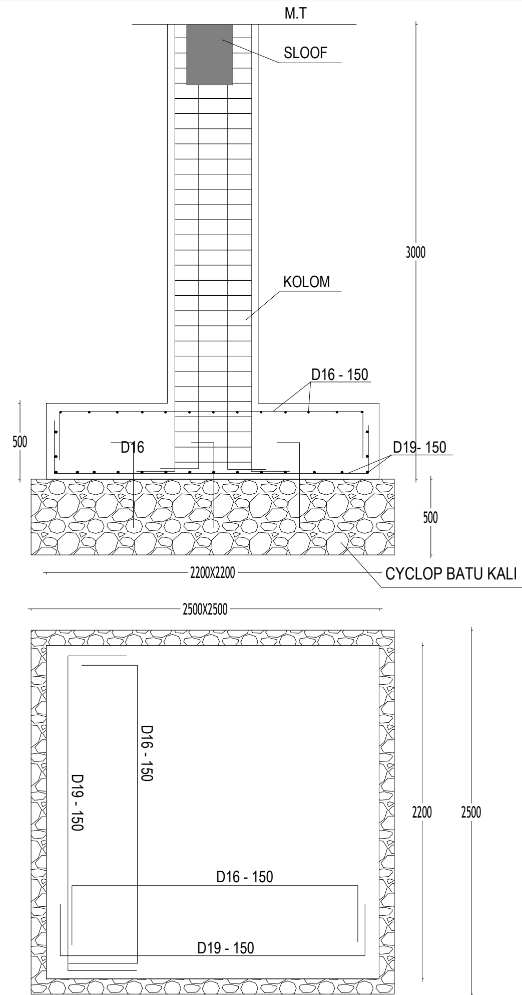
DETAIL FONDASI F1
