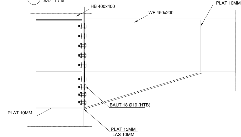
DETIL B2 KE KOLOM SKALA 1 : 15
