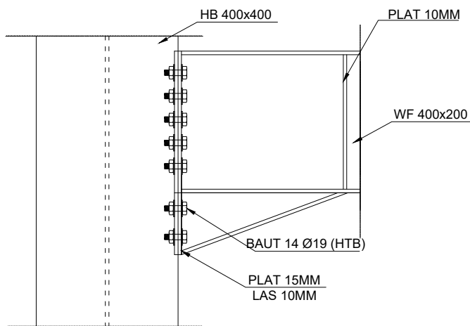
DETIL B3 KE KOLOM SKALA 1 : 15
