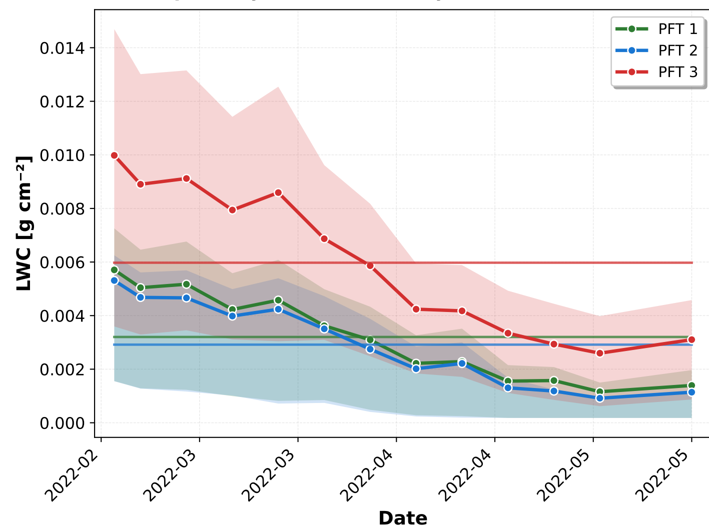
(d) Temporal Dynamics of LWC by PFT
