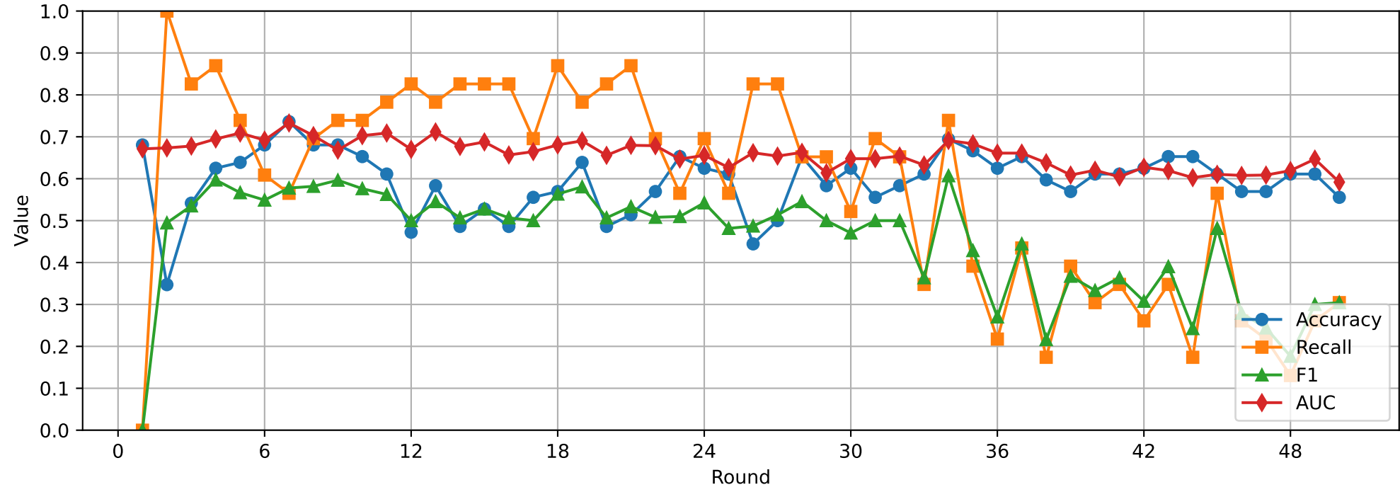
Arkansas Metrics Per Round
