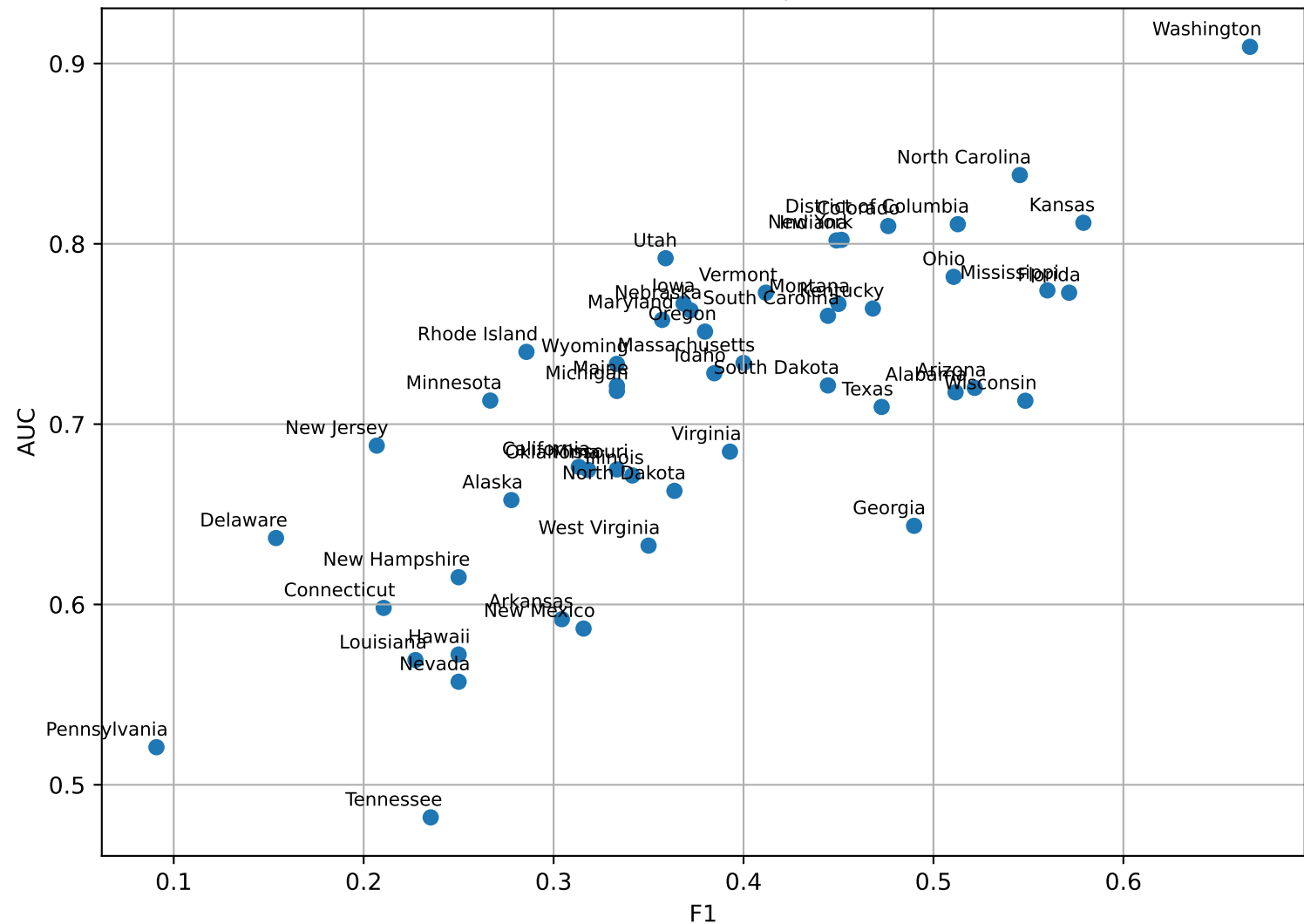
F1/AUC Scatterplot
