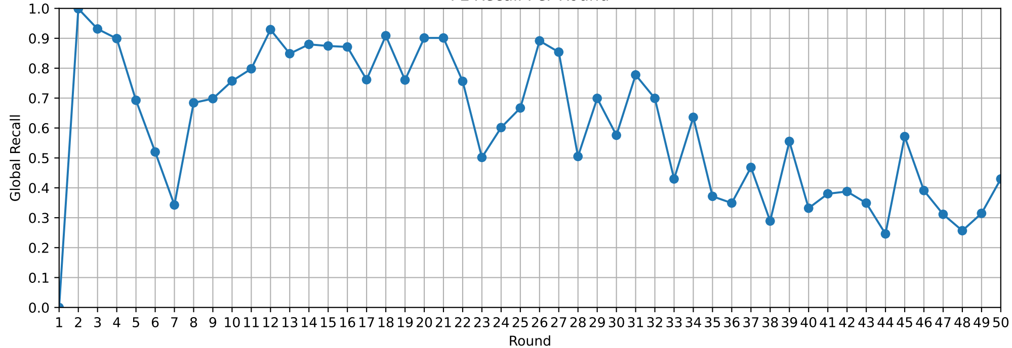
FL Recall Per Round
