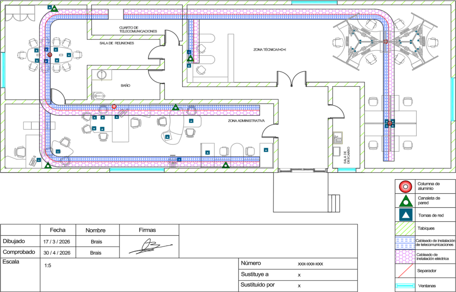
Plano de planta con la canalización y ubicación de las tomas
