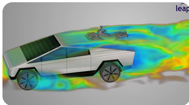
Figura 5.1: Análisis aerodinámico sobre Cybertruck Tesla Motors inc.
