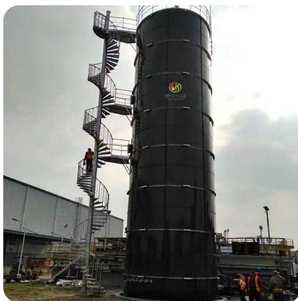
Figura 5.3: Biodigestor para producción de biogas.
