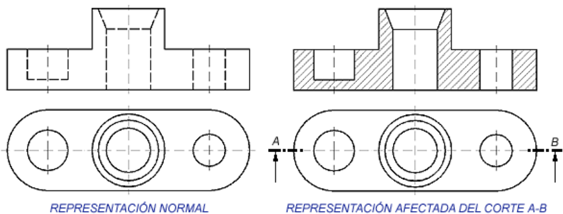
Figura 1.19: Corte.
