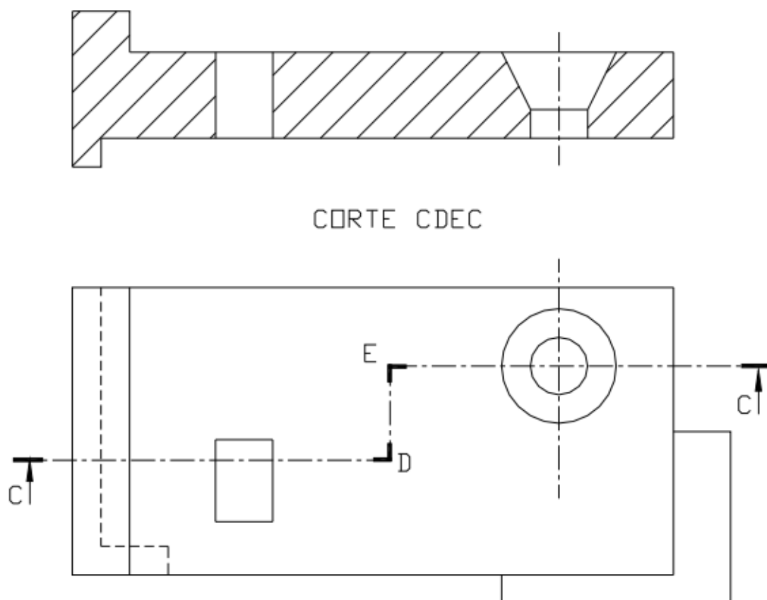
Figura 1.22: Corte quebrado.
