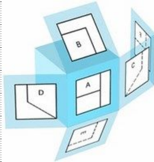
Figura 1.9: Sistema Americano
