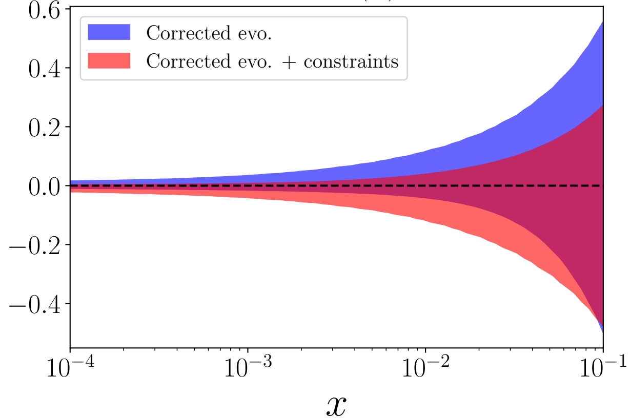
x\Delta u^+(x)
