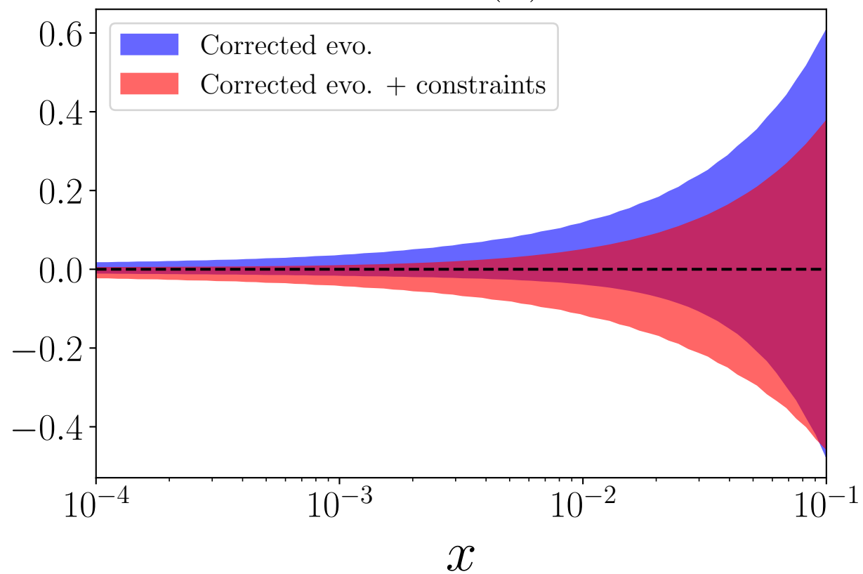
x\Delta s^+(x)
