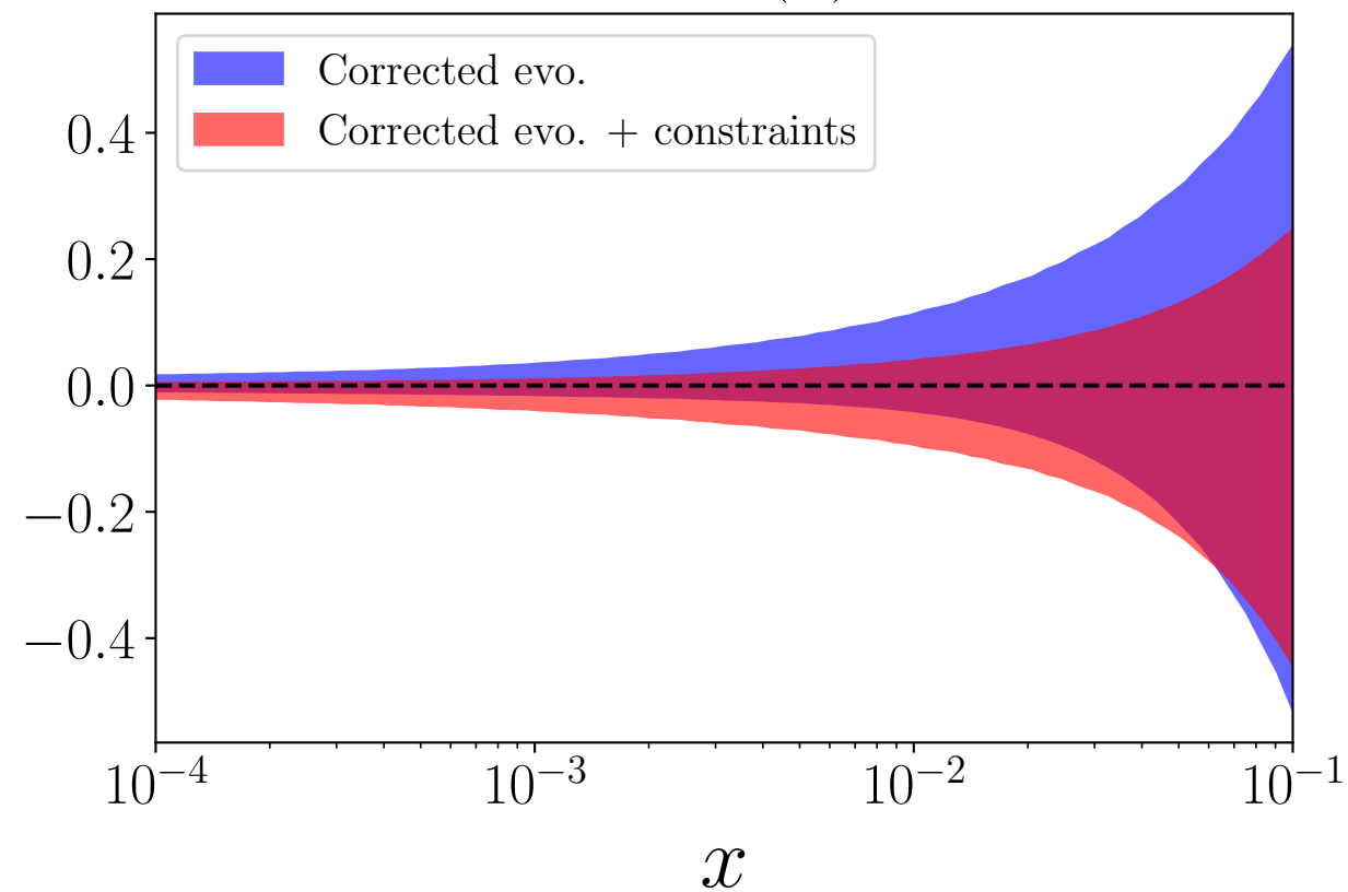
x\Delta d^+(x)
