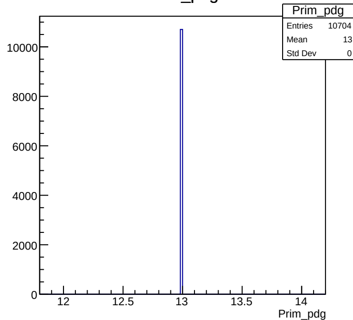
Prim_pdg
