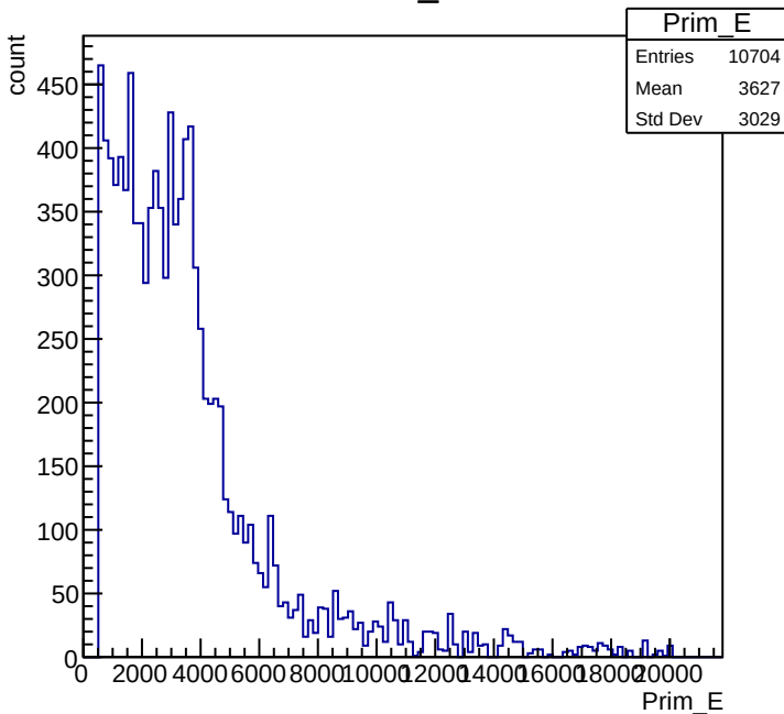
Prim_E
