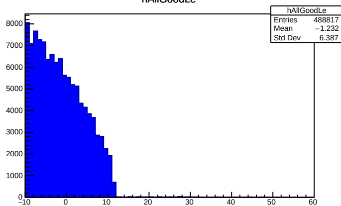
hAllGoodLe
