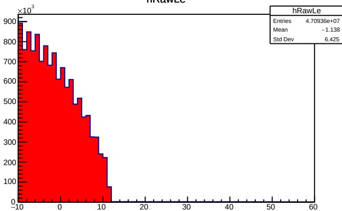
hRawLe
