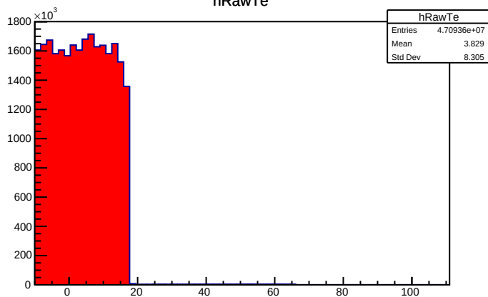
hRawTe
