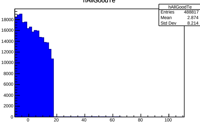
hAllGoodTe
