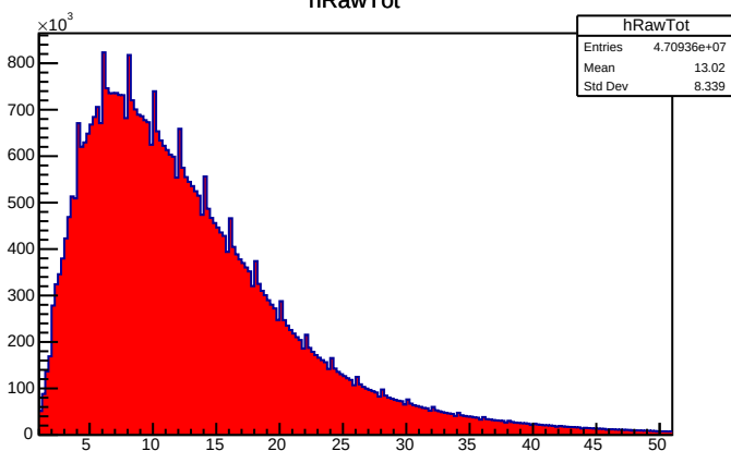
hRawTot
