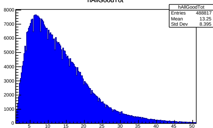
hAllGoodTot
