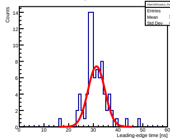
Bar 100, Paddle 1604
