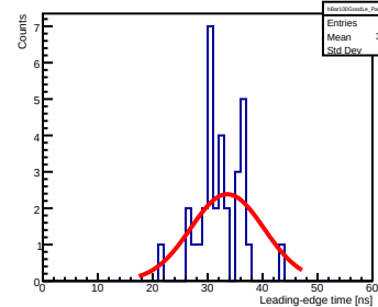
Bar 100, Paddle 1612
