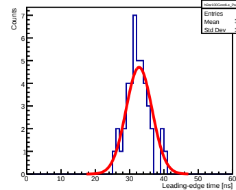
Bar 100, Paddle 1608
