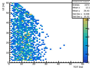
Good LE vs TOT (Paddle 476)
