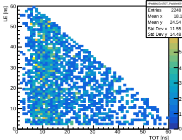
Good LE vs TOT (Paddle 473)
