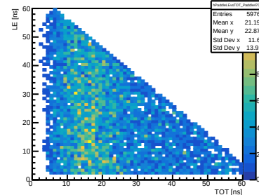
Good LE vs TOT (Paddle 474)
