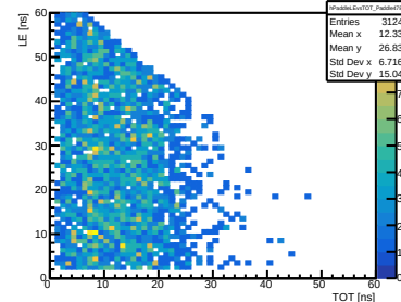
Good LE vs TOT (Paddle 478)
