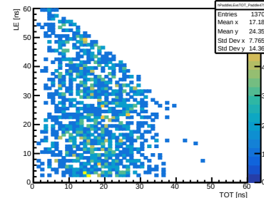
Good LE vs TOT (Paddle 479)
