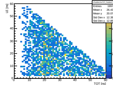
Good LE vs TOT (Paddle 475)
