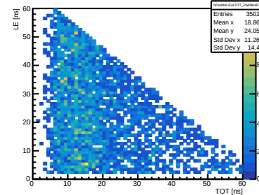
Good LE vs TOT (Paddle 471)
