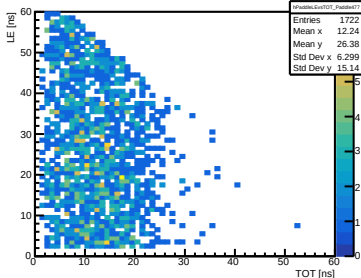
Good LE vs TOT (Paddle 477)
