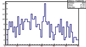
LE (Paddle 492)
