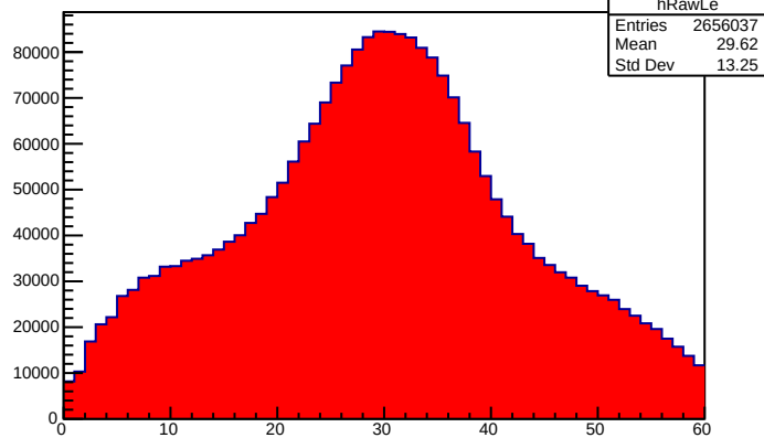
hRawLe
