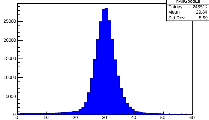
hAllGoodLe
