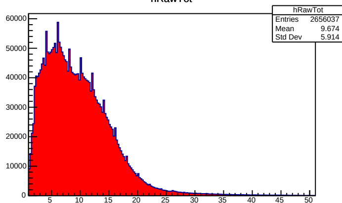
hRawTot
