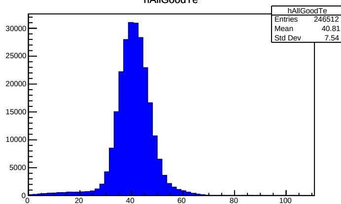
hAllGoodTe
