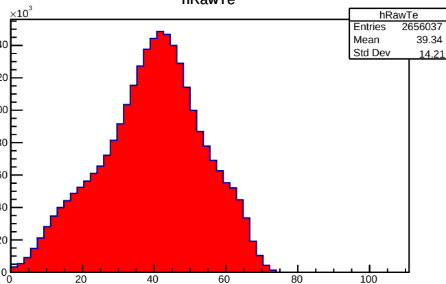
hRawTe
