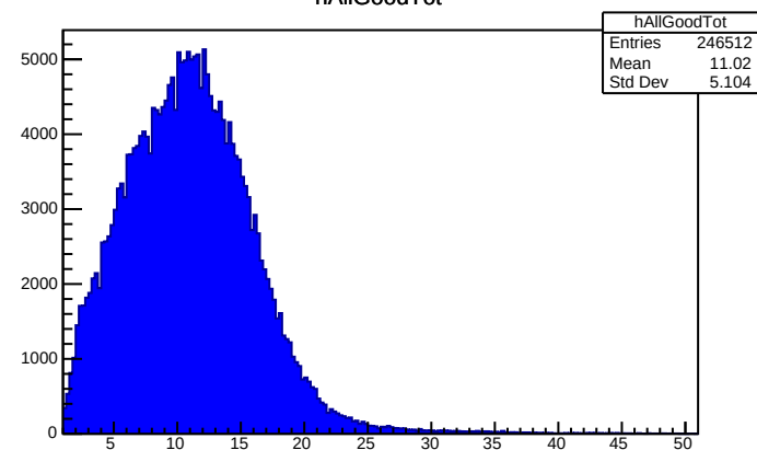
hAllGoodTot
