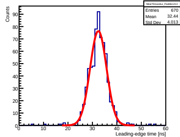
Bar 75, Paddle 1213
