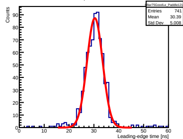
Bar 75, Paddle 1215
