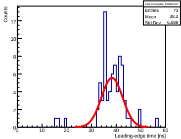
Bar 144, Paddle 2317
