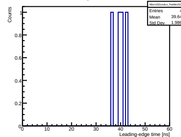
Bar 145, Paddle 2327
