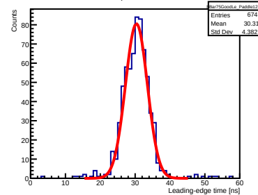
Bar 75, Paddle 1215
