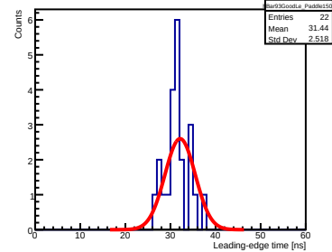
Bar 93, Paddle 1501
