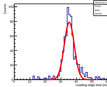
Bar 62, Paddle 1006
