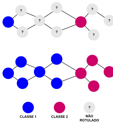
Figura 17.7: Processo de propagação de rótulos em um grafo. Partindo de poucos exemplos rotulados (topo), o algoritmo propaga os rótulos aos nós vizinhos não rotulados, mudando esses rótulos até que um equilíbrio seja atingido (base).
