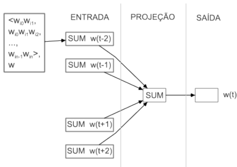
Figura 10.8: Arquitetura FastText-CBOW.
