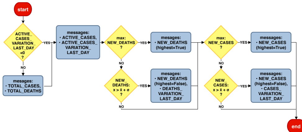
Figura 13.7: Módulo de Seleção de Conteúdo do robô-jornalista “CoronaReporter”.
