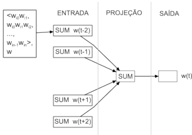
Figura 10.8: Arquitetura FastText-CBOW.
