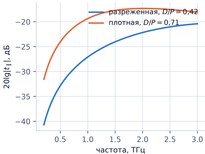
Канал подавления |t_{\parallel}| , дБ
