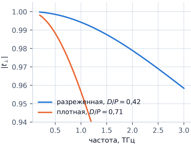
Канал пропускания |t_{\perp}|
