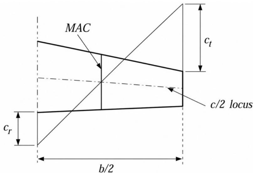
Figura 4.3: Metodo grafico per la corda media aerodinamica.
