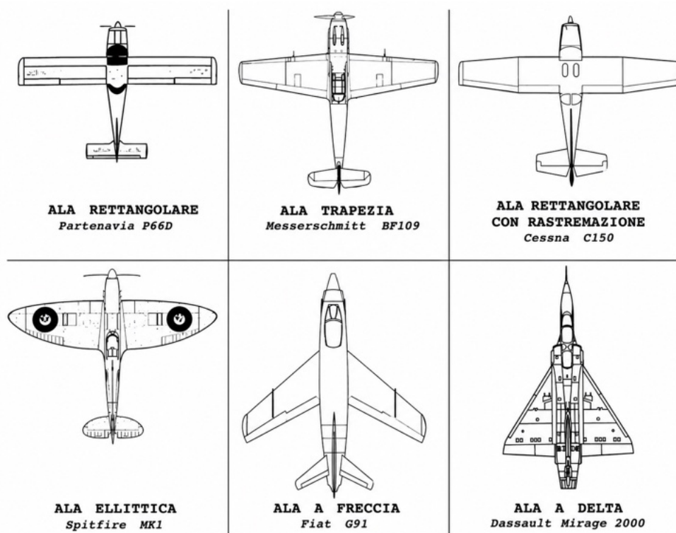
Figura 4.1: Forme in pianta dell'ala con esempi storici.
