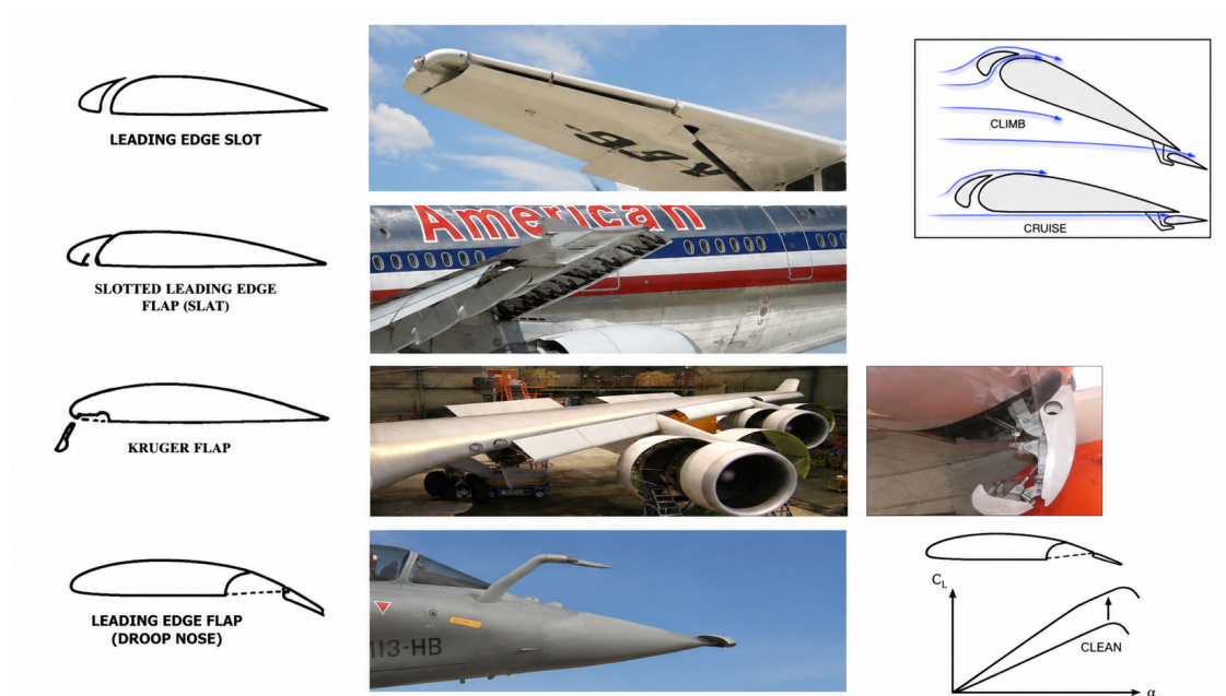
Figura 3.2. Esempi reali: leading edge slot fisso su velivolo STOL (aperto in salita, chiuso in crociera); slat dell'A300 e del Mirage 2000; Kruger flap del B747; droop nose su velivolo da combattimento.
