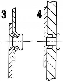
Schema del tipo di giunzione (dal manuale, Tab. 3)
