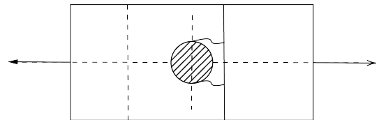
Fig. 4 — Tranciamento al bordo libero (Modo IV)
