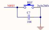
RST复位-按键
