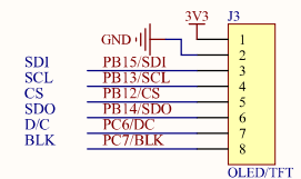
OLED/TFT液晶接口
