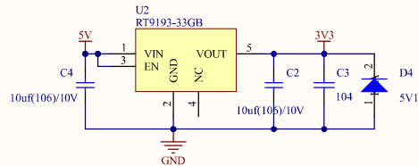
系统供电稳压
