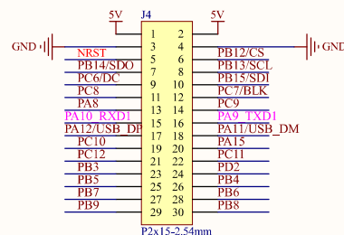
通用I/O接口
