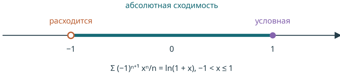
Рис. 3.3: Для ряда логарифма: расходимость при -1 , абсолютная сходимость внутри и условная при 1 .
