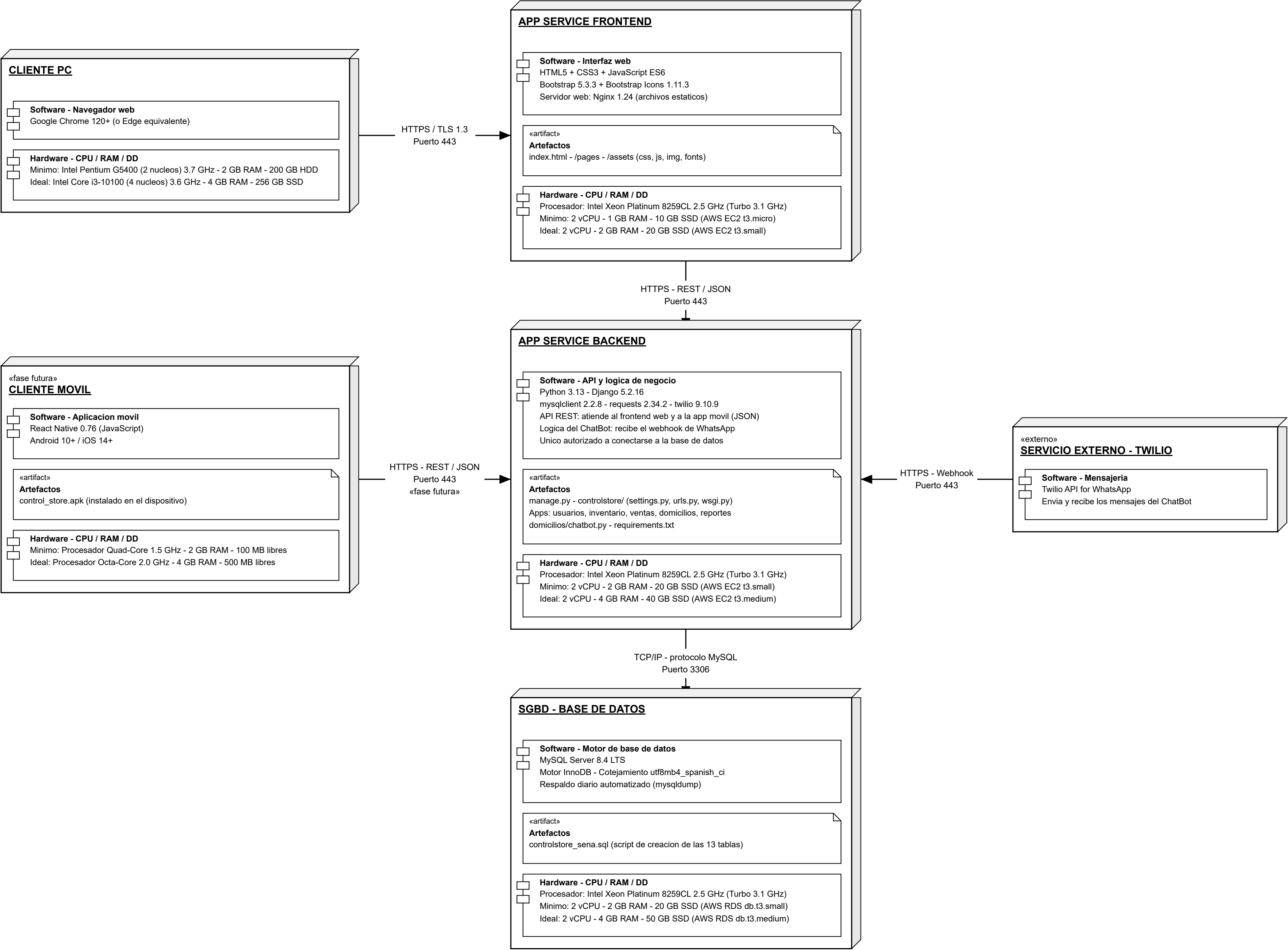
Diagrama de despliegue - Control Store | Autoservicio Ayuelal
