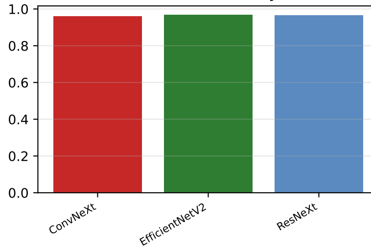
F1 (macro)
