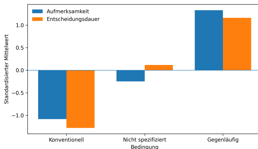
Abbildung 1: Mittlere subjektive Aufmerksamkeit und Entscheidungsdauer in den drei experimentellen Bedingungen. Die beiden Kennwerte sind zur Vergleichbarkeit standardisiert dargestellt.
