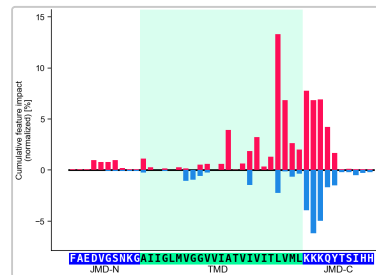
CPPPlot.profile · SHAP
