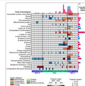
CPPPlot.feature_map · SHAP
