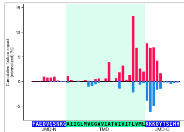
CPPPlot.profile · SHAP
