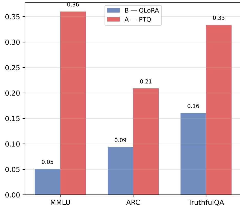
ECE
