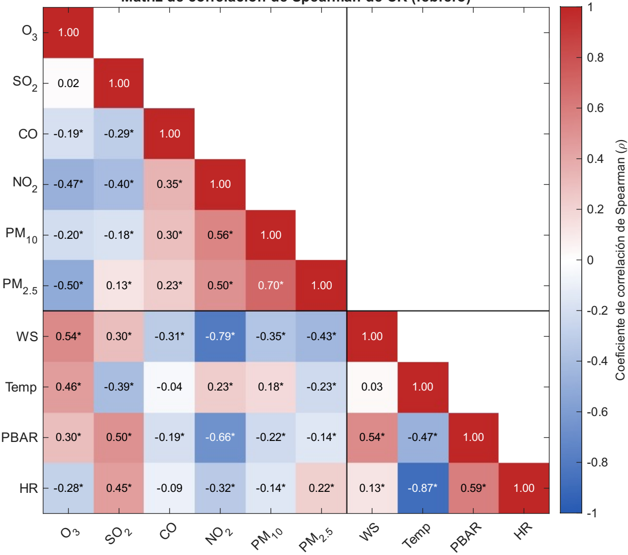
Matriz de correlación de Spearman de CR (febrero)
