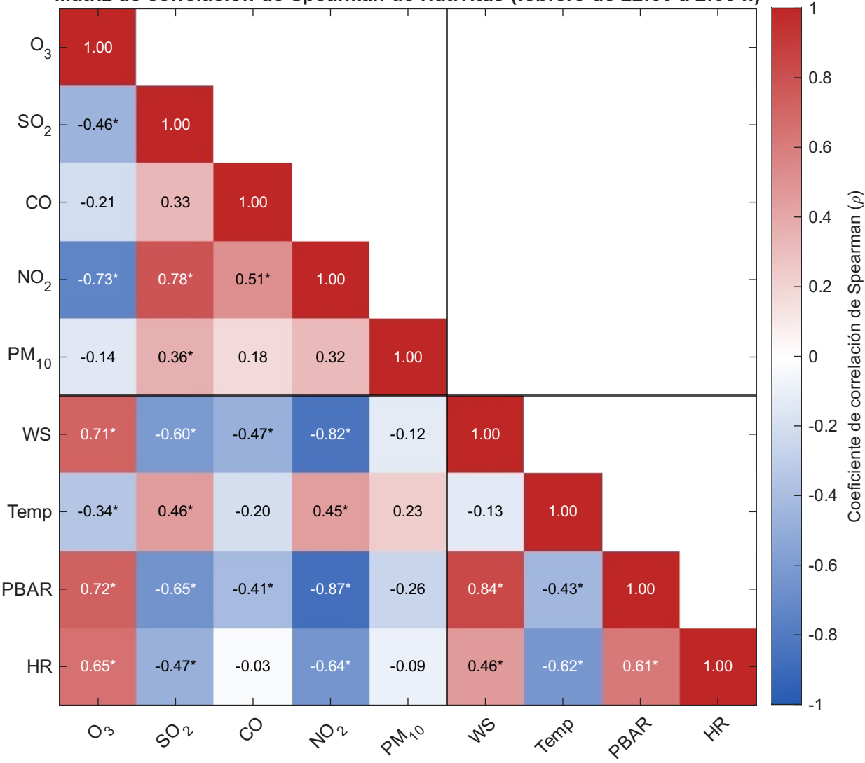
Matriz de correlación de Spearman de Nativitas (febrero de 22:00 a 2:00 h)
