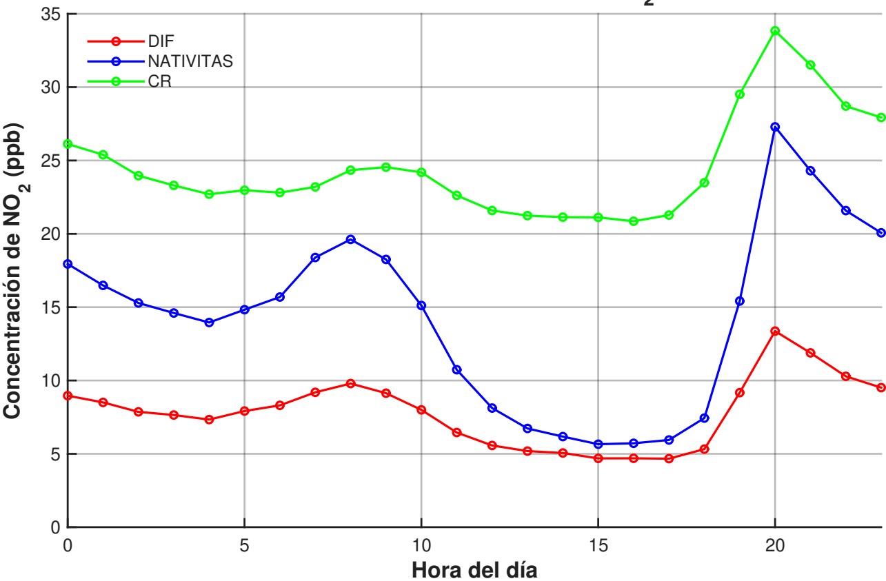
Variación de la concentración horaria de NO 2 en Salamanca
