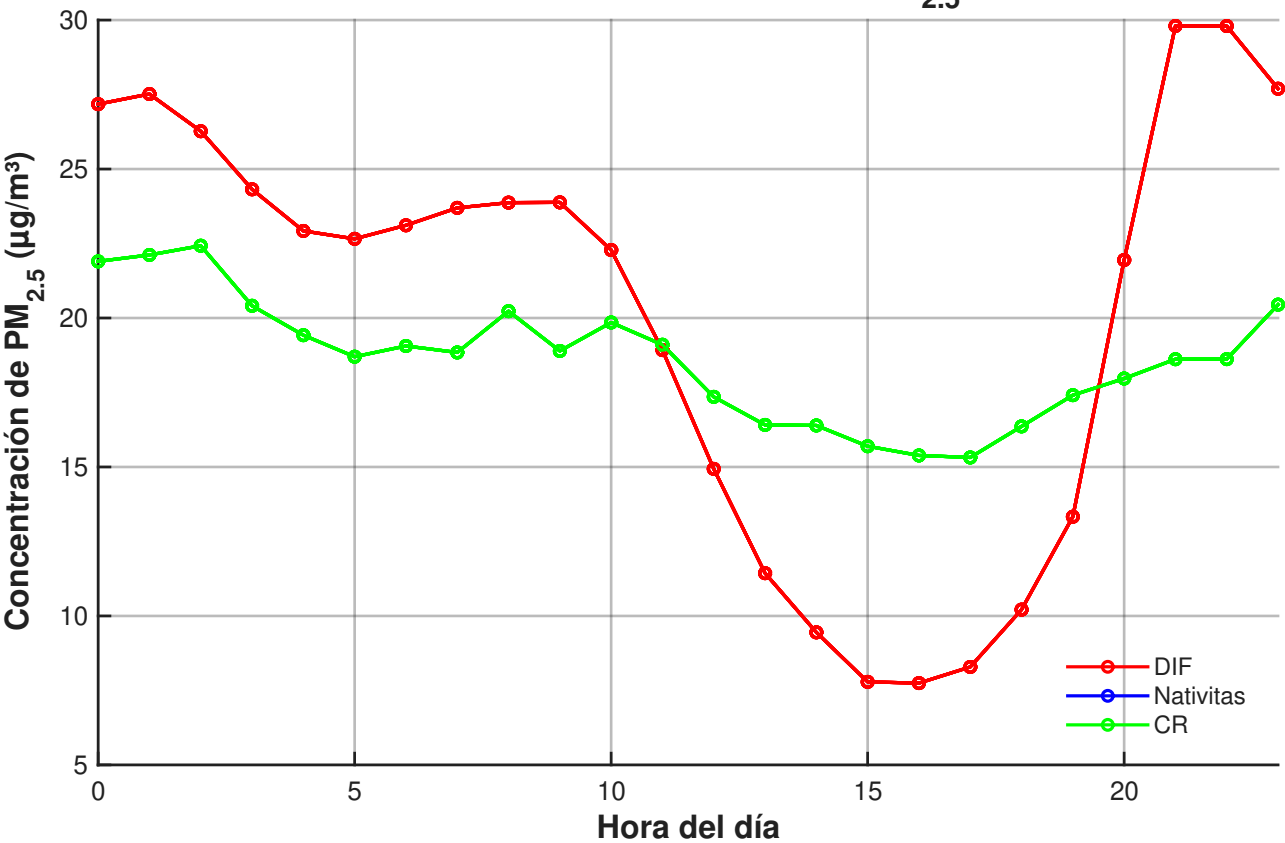
Variación de la concentración horaria de \text{PM}_{2.5} en Salamanca
