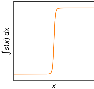
MEDT ( \varepsilon > 0 )
