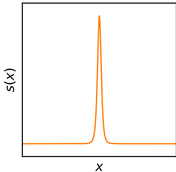
MEDT ( \varepsilon > 0 )
