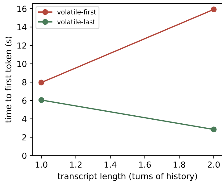
Prefill vs. prompt layout
