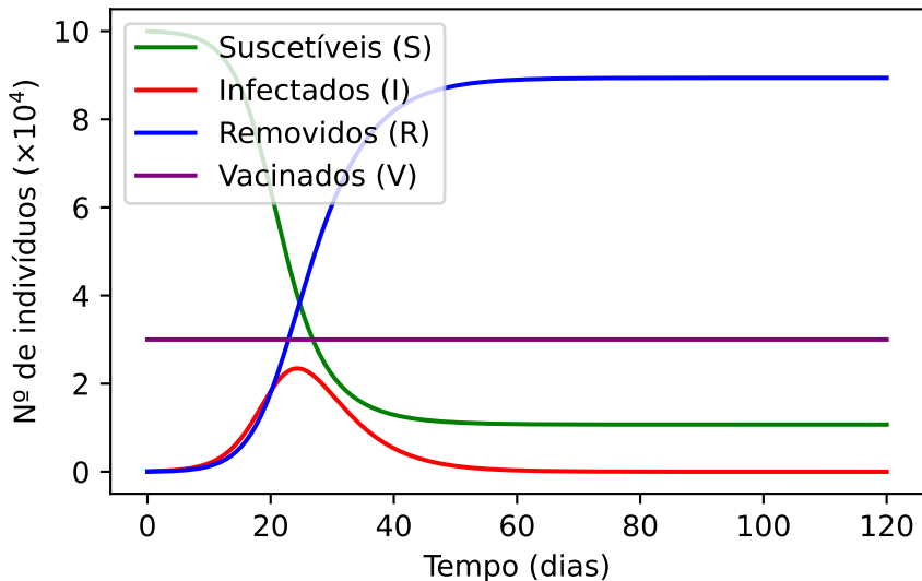
Figura 7: Simulação do modelo SIRV, com \rho = 0.3
