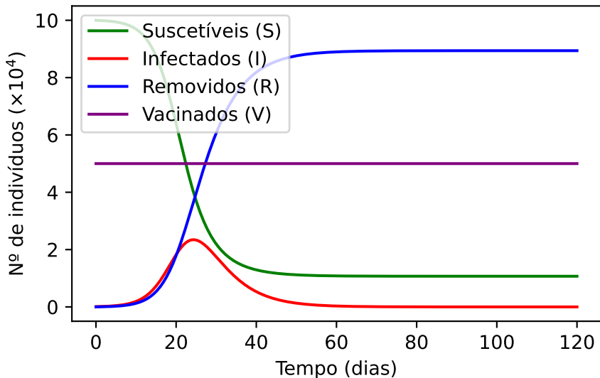
Figura 8: Simulação do modelo SIRV, com \rho = 0.5
