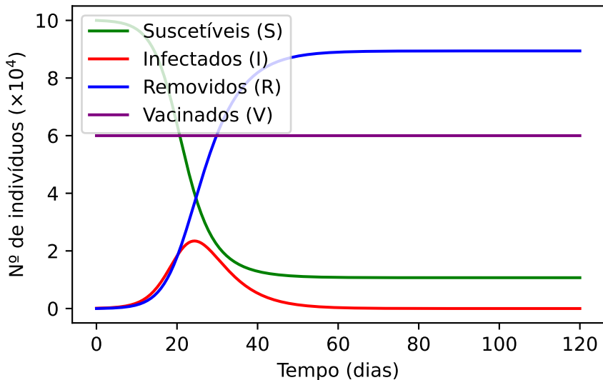
Figura 9: Simulação do modelo SIRV, com \rho = 0.6
