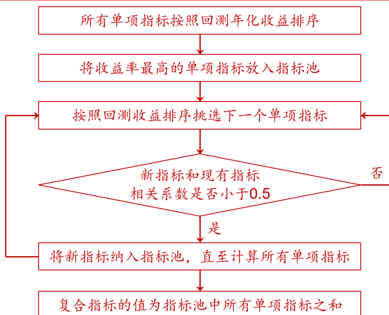
图表40: 复合景气度指标构建流程
