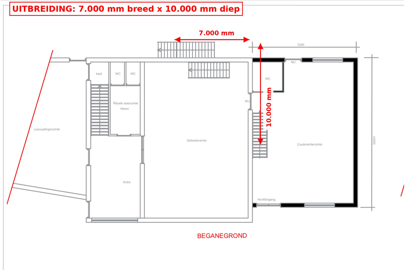
Figuur 6 - C1 - Nieuwe uitbreiding begane grond met duidelijke maatvoering
