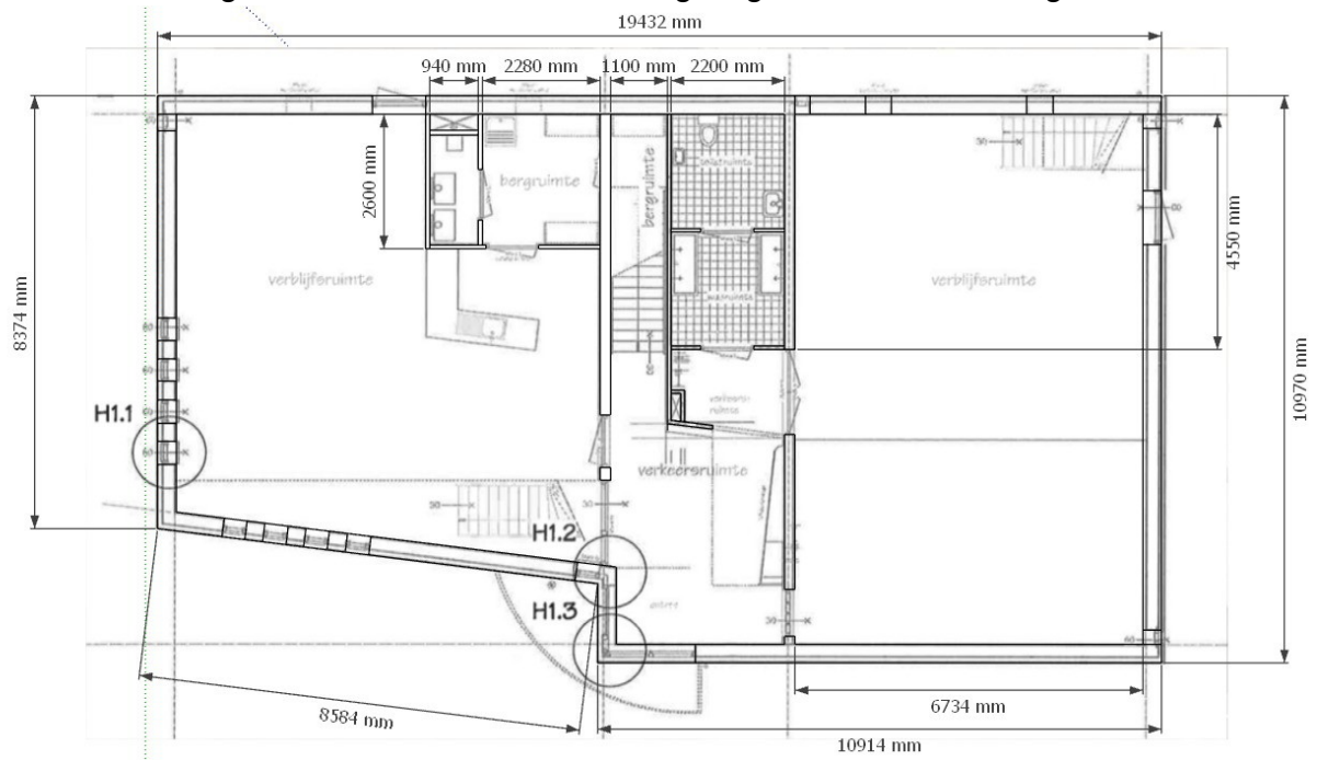
B1 - Bestaande situatie begane grond met maatvoering.
