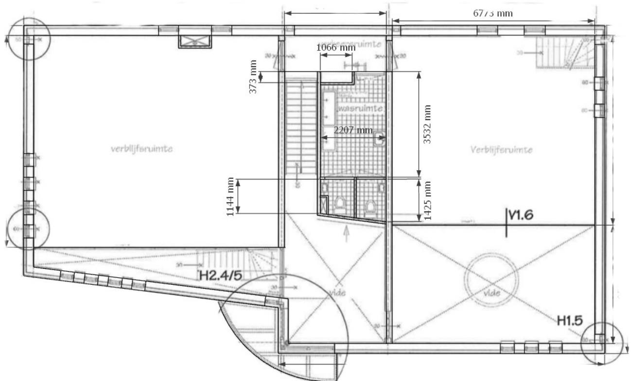
B2 - Bestaande situatie verdieping met maatvoering.
