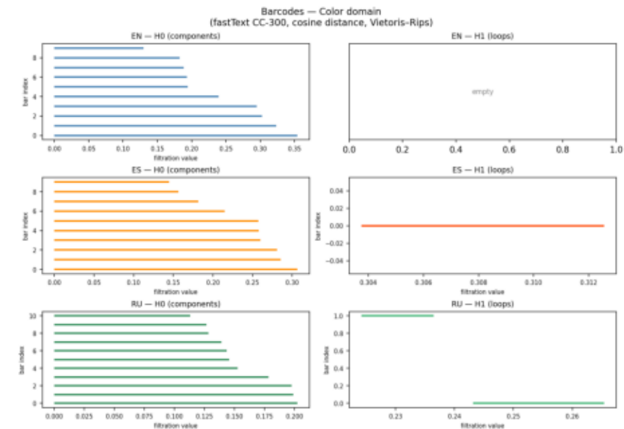
B barcodes — Color (EN / ES / RU)
