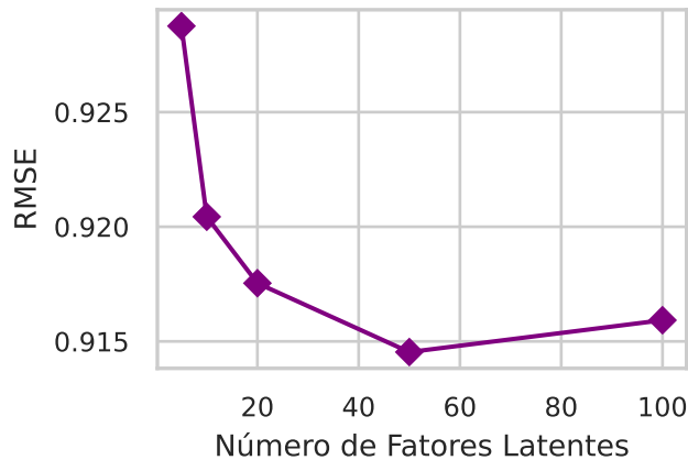
SVD++
