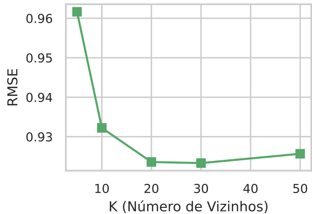
SVD++
