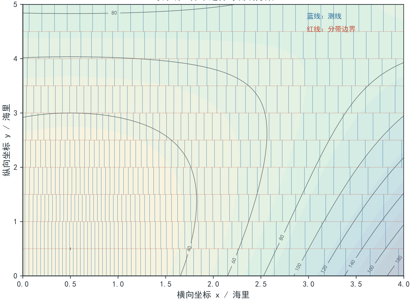
等深线、分带边界与测线方案
