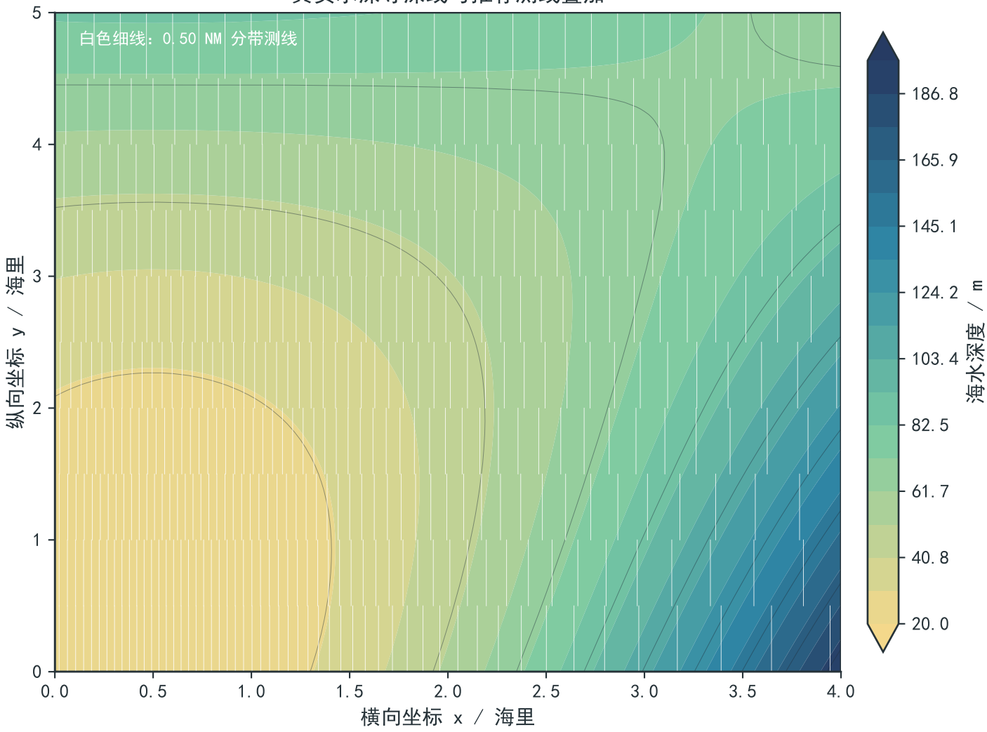
真实水深等深线与推荐测线叠加
